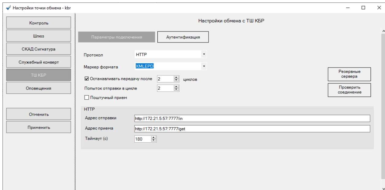
Рис 1а. Настройки обмена ТШ КБР для ПП АРМ КБР-Н (Протокол HTTP, тестовый контур)
