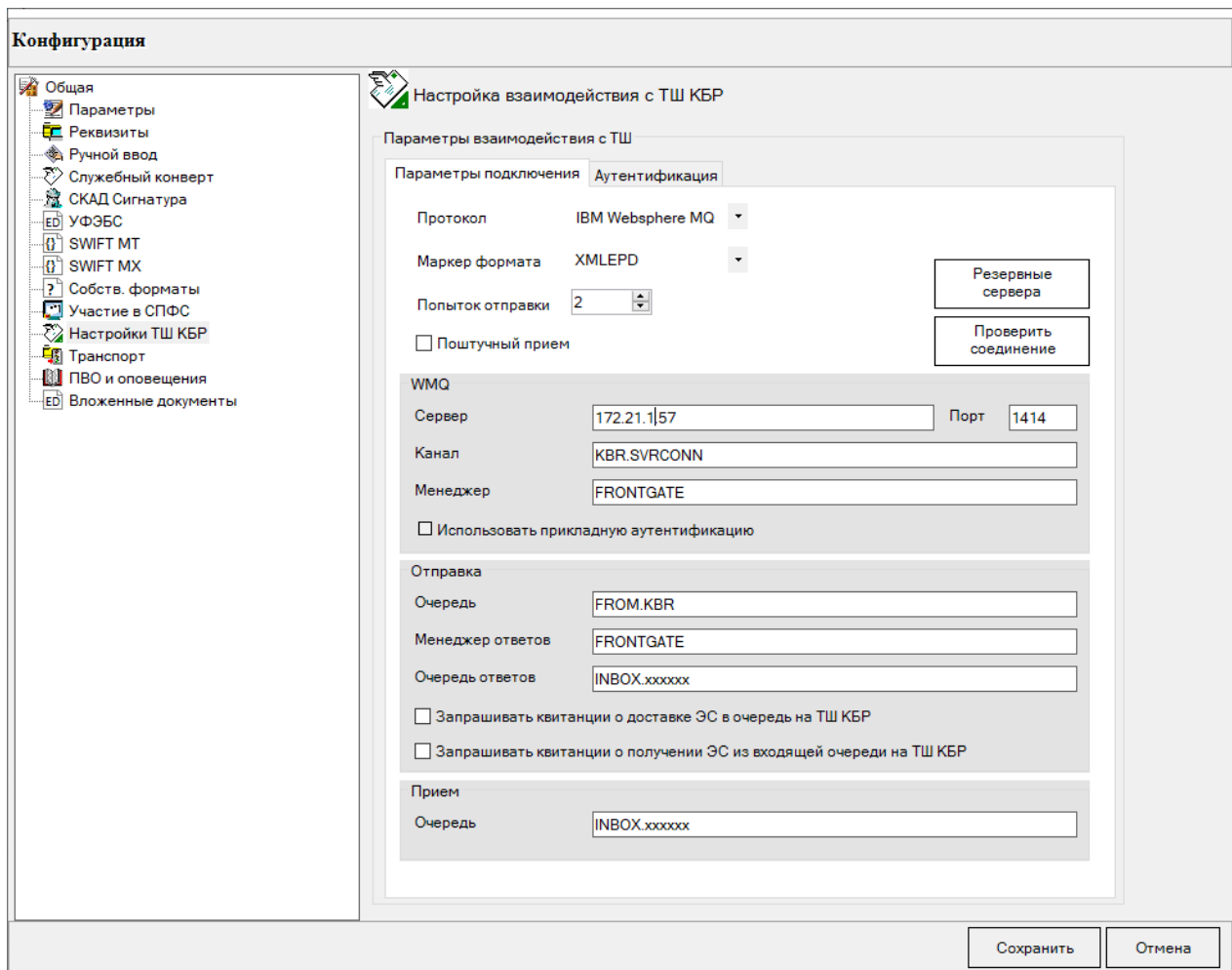
Рис 46. Настройки взаимодействия с ТШ КБР для ПП АРМ КБР-СПФС (Протокол MQ, промышленный контур)
