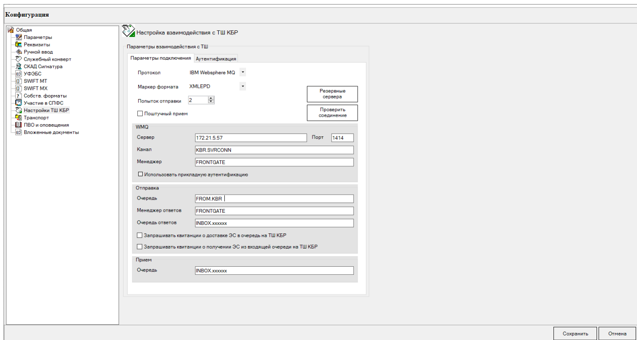
Рис 26. Настройки взаимодействия ТШ КБР для ПП АРМ КБР-СПФС (Протокол MQ, тестовый контур)
