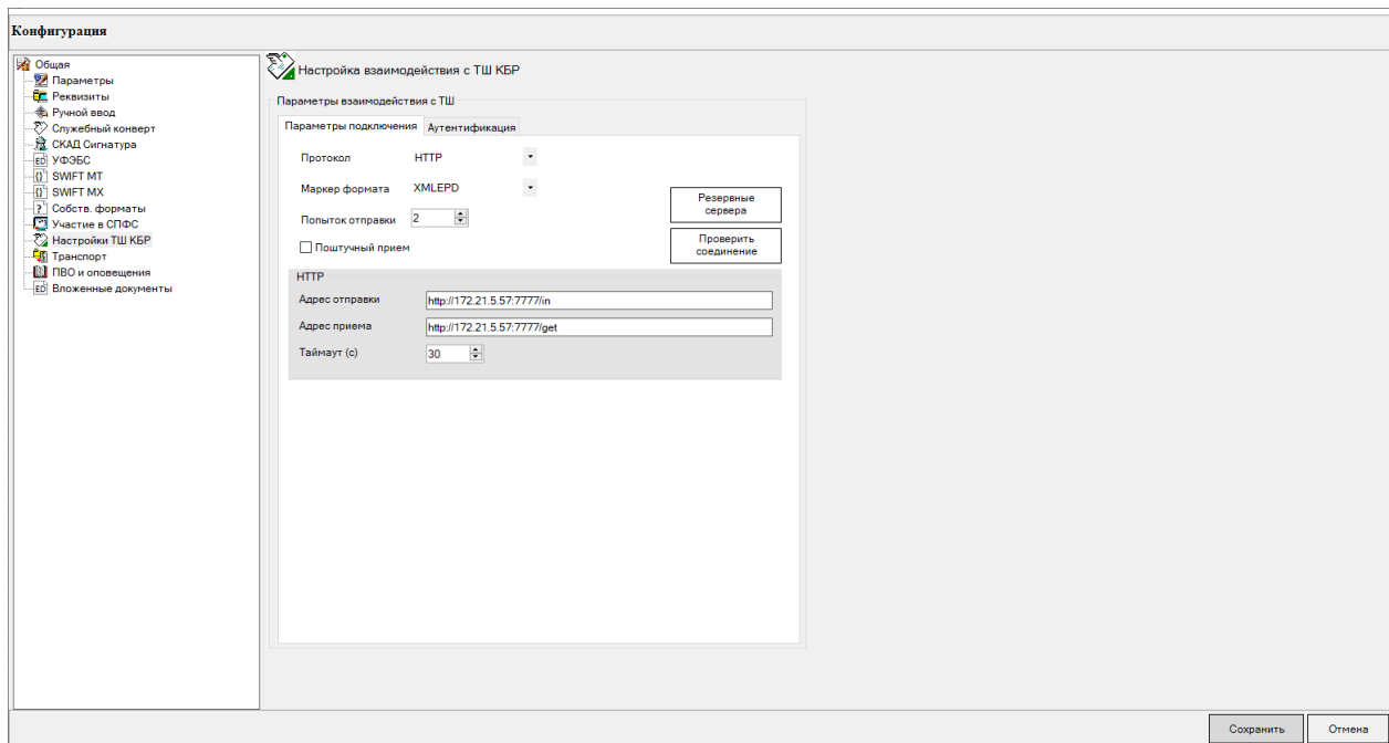
Рис 1а. Настройки обмена ТШ КБР для ПП АРМ КБР-Н (Протокол HTTP, тестовый контур)
