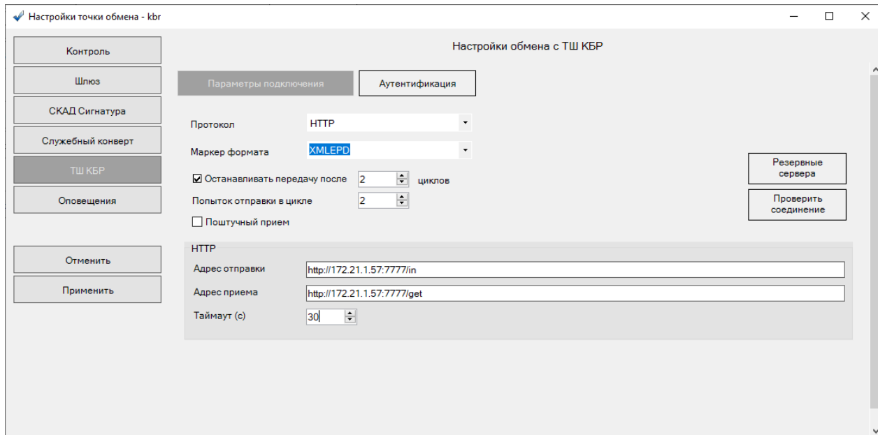
Рис 3а. Настройки обмена ТШ КБР для ПП АРМ КБР-Н (Протокол HTTP, промышленный контур)
