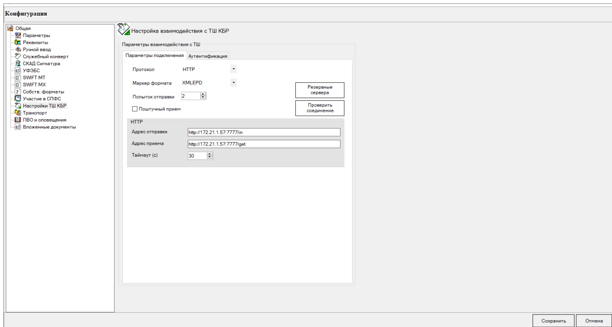
Рис 3б. Настройки взаимодействия с ТШ КБР для ПП АРМ КБР-СПФС (Протокол HTTP, промышленный контур)
